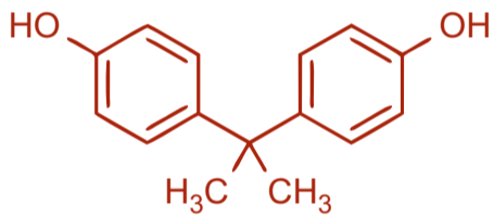
bisphenol A
